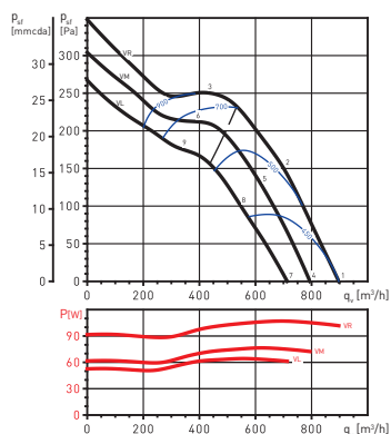
TD EVO 200
